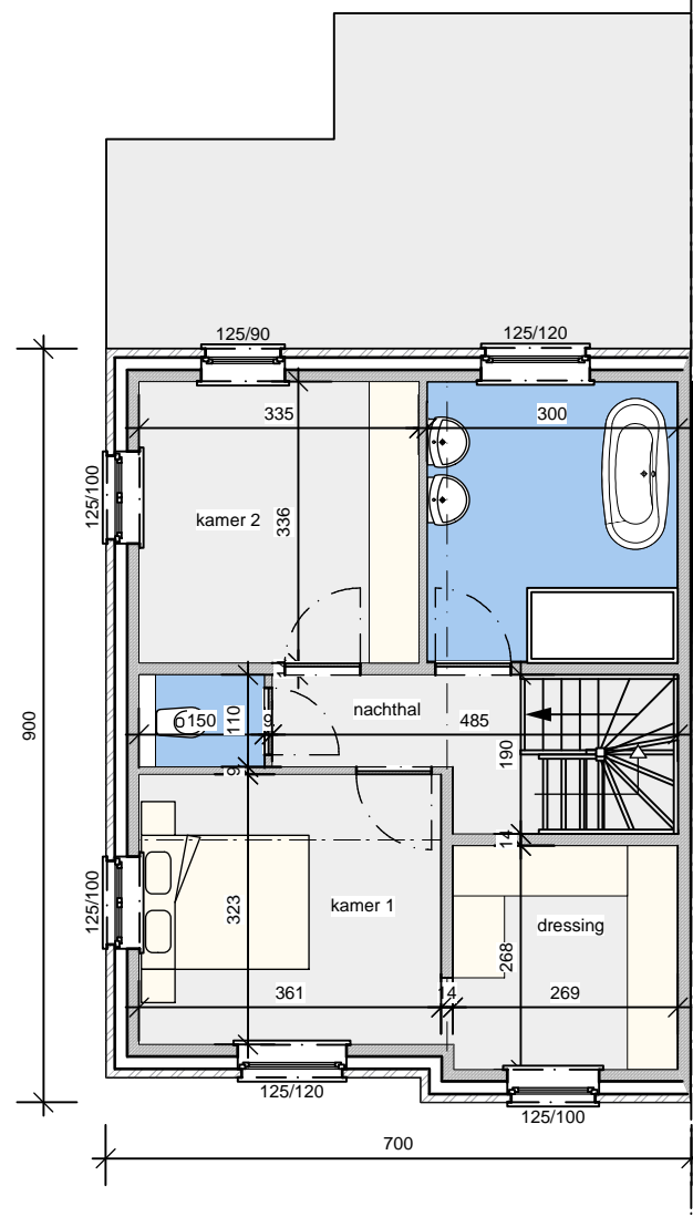
verdieping 61 m 2
