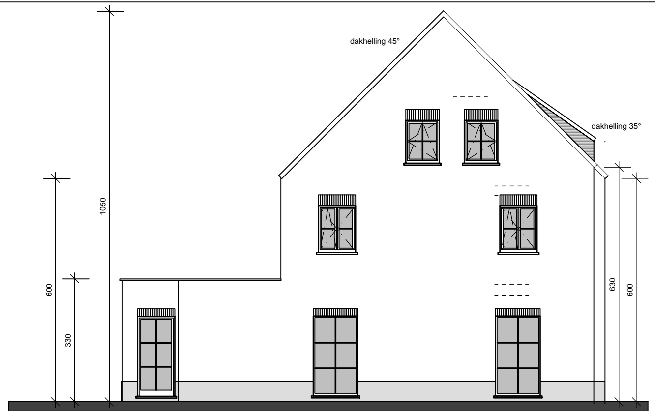
rechtergevel
