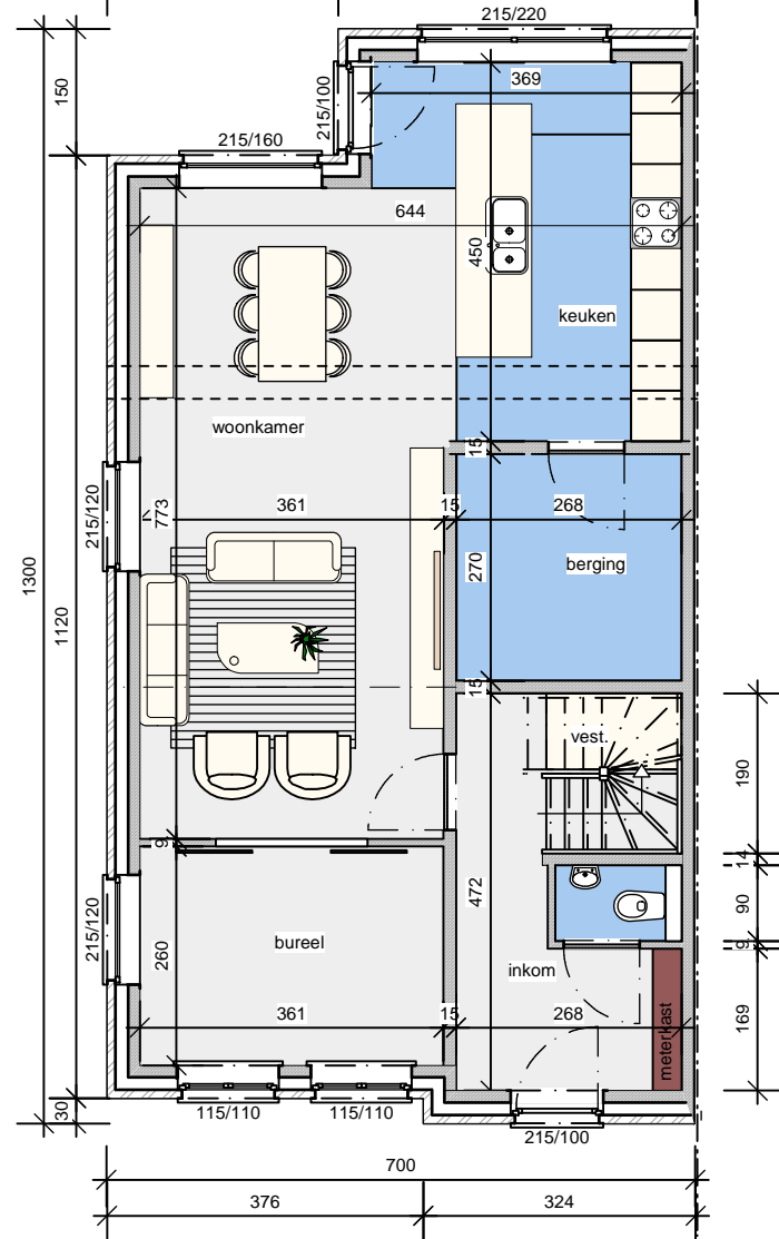
gelijkvloers 85 m 2
